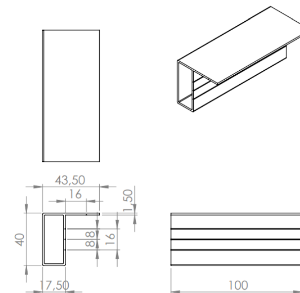
Profil imbinare 40 mm
