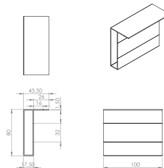
Profil imbinare 80 mm
